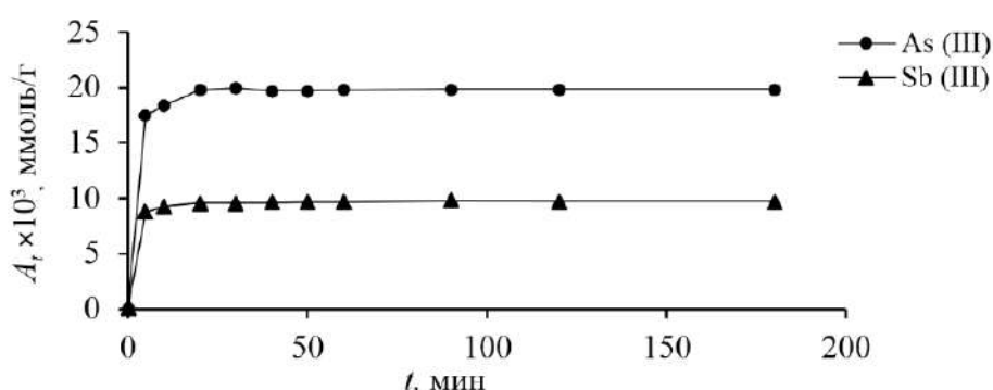
Кинетические кривые сорбции ионов As (III) и Sb (III) на ММ:КПАВ:Fe 3 O 4 .
