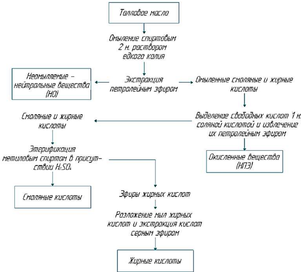
Рис. 1. Принципиальная схема группового анализа сырого таллового масла
