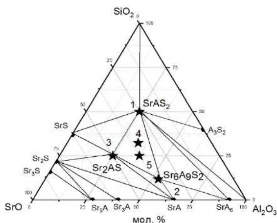
Рис. 1. Диаграмма треугольников сосуществующих фаз системы SrO-Al 2 O 3 -SiO 2 в субсолидусной области при температуре 1350 °C [5], ★ — синтезированные образцы
