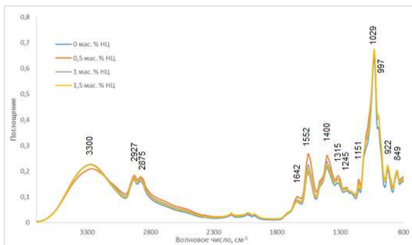
Рис. 1. ИК-спектры образцов хитозановых плёнок, армированных nanoцеллюлозой
