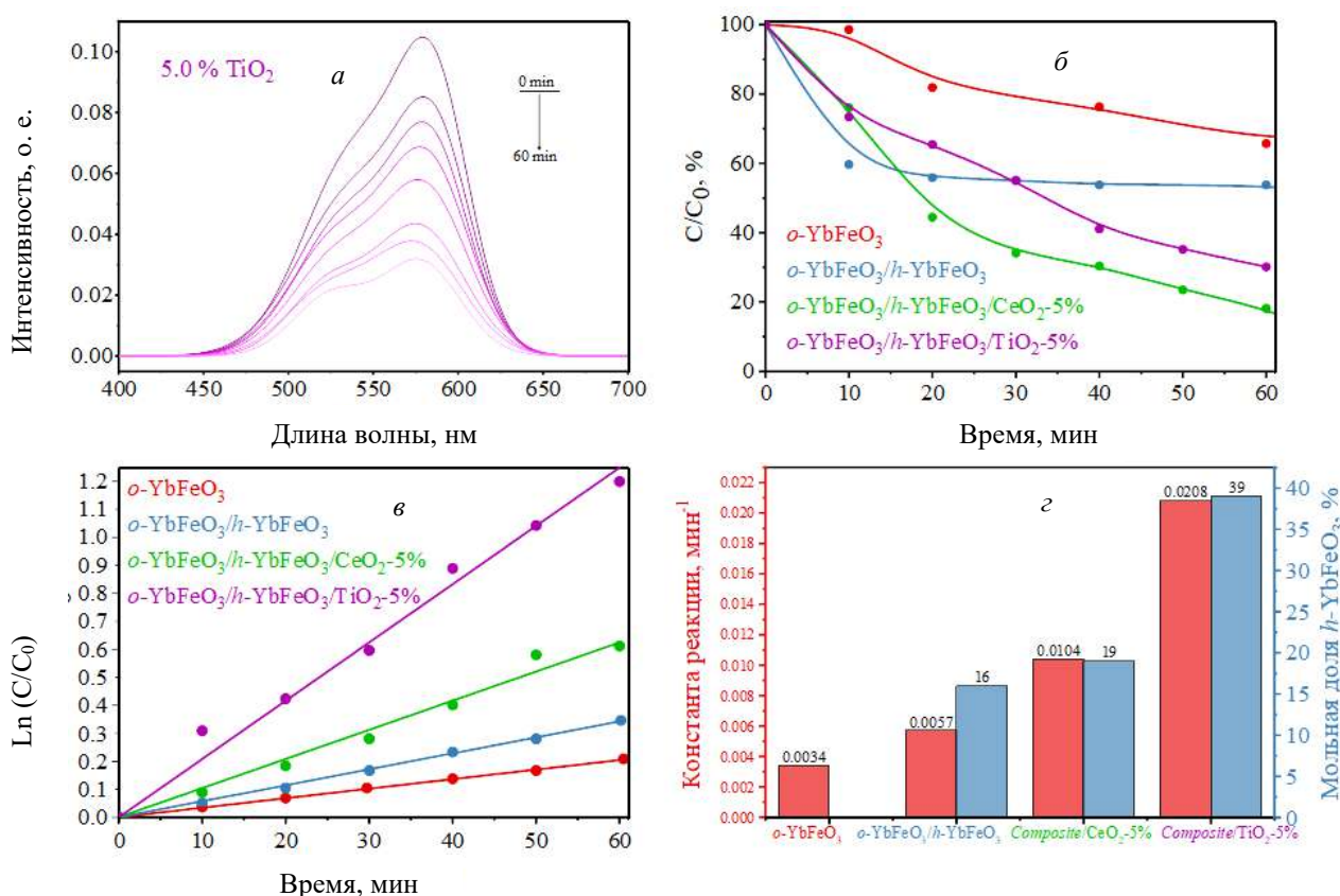
Рис. 3. Результаты кинетических исследований процесса фотофентоноподобного разложения метилового фиолетового в присутствии \text{YbFeO}_3/h\text{-YbFeO}_3/\text{MO}_2 ( M = \text{Ce}, \text{Ti} )
