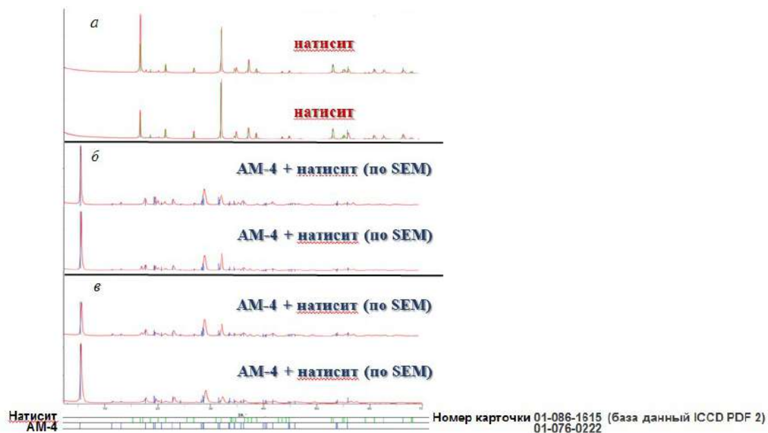
Рис. 1. Результаты РФА синтезированных фаз на основе разных источников титана: а — \text{TiCl}_4 ; б — \text{TiCl}_3 ; в — (\text{NH}_4)_2\text{TiO}(\text{SO}_4)_2 \cdot \text{H}_2\text{O}
