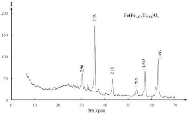
Рис. 1. Дифрактограмма титаномагнетита
