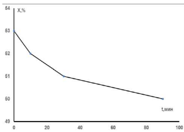
Рис. 4. Выход летучих веществ продуктов низкотемпературного ТО для ЭП категории В в зависимости от продолжительности процесса
