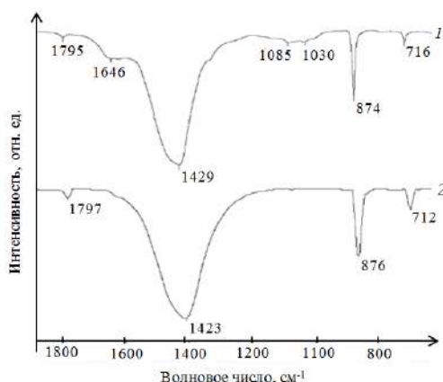
Рис. 1. Фрагмент спектров инфракрасного поглощения дефеката (1) и кальцита (2)
