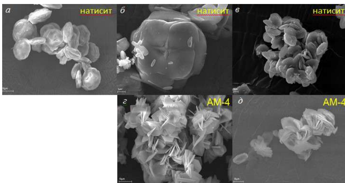
Рис. 2. Результаты электронно-зондовой микроскопии продуктов синтеза, полученных на основе разных источников титана: а — \text{TiCl}_4 ; б , в — \text{TiCl}_3 ; д — соль СТА
