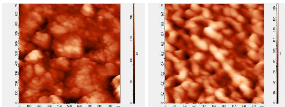
Рис. 2. АСМ-изображения поверхности образца литейного экспериментального сплава: слева — после анодирования в универсальном электролите ( j_a = 25 мА/см 2 , t_a = 90 мин); справа — после гидротермальной обработки
