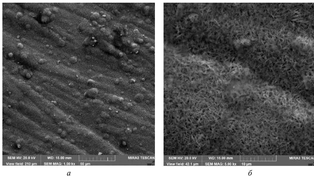
Рис. 2. Микроструктура покрытий сплава цинк-никель после обработки в растворе хроматирования и нанесения ПВС при увеличении 1,0 кх (а) и 5,0 кх (б)
