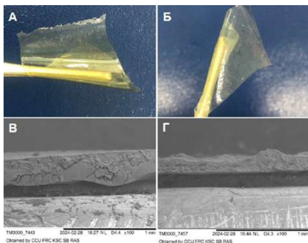
Рис. 2. Микрофотографии композитной плёнки без добавления (А) и с добавлением 1,5 мас. % nanoцеллюлозы (Б), среза плёнки без добавления (В) и с добавлением 1,5 мас. % nanoцеллюлозы (Г)
