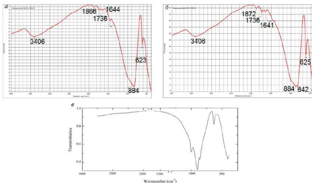
Рис. 3. Результаты ИК-спектроскопии натасита:
