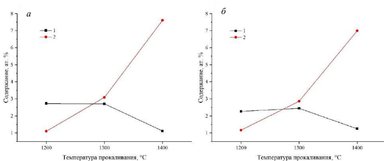
Рис. 3. Содержание Се в гафноне (1) и Hf в церианите (2) в зависимости от температуры прокаливания МА-смесей: а — \text{SiO}_2 реактивный; б — \text{SiO}_2 из шлака
