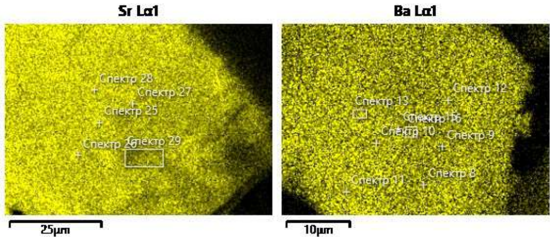
Рис. 2. Распределение элементов Sr и Ba по поверхности стронций- и бариймодифицированных ГАП
