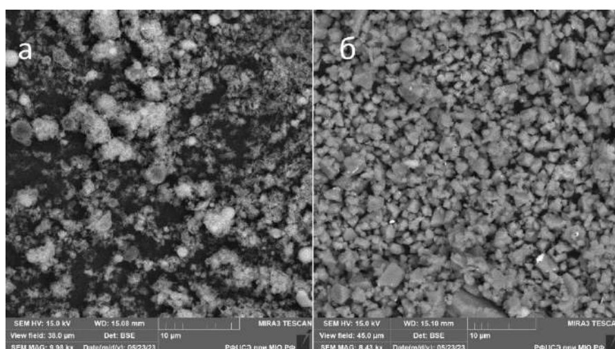
Рис. 4. Фотографии микроструктуры порошков алюмомагниевого шпинели с добавкой, полученных первым (а) и вторым (б) методами
