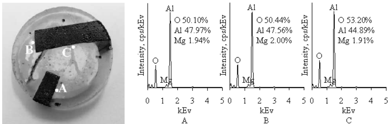
Внешний вид и спектры характеристического излучения в различных участках (A, B, C) образца
